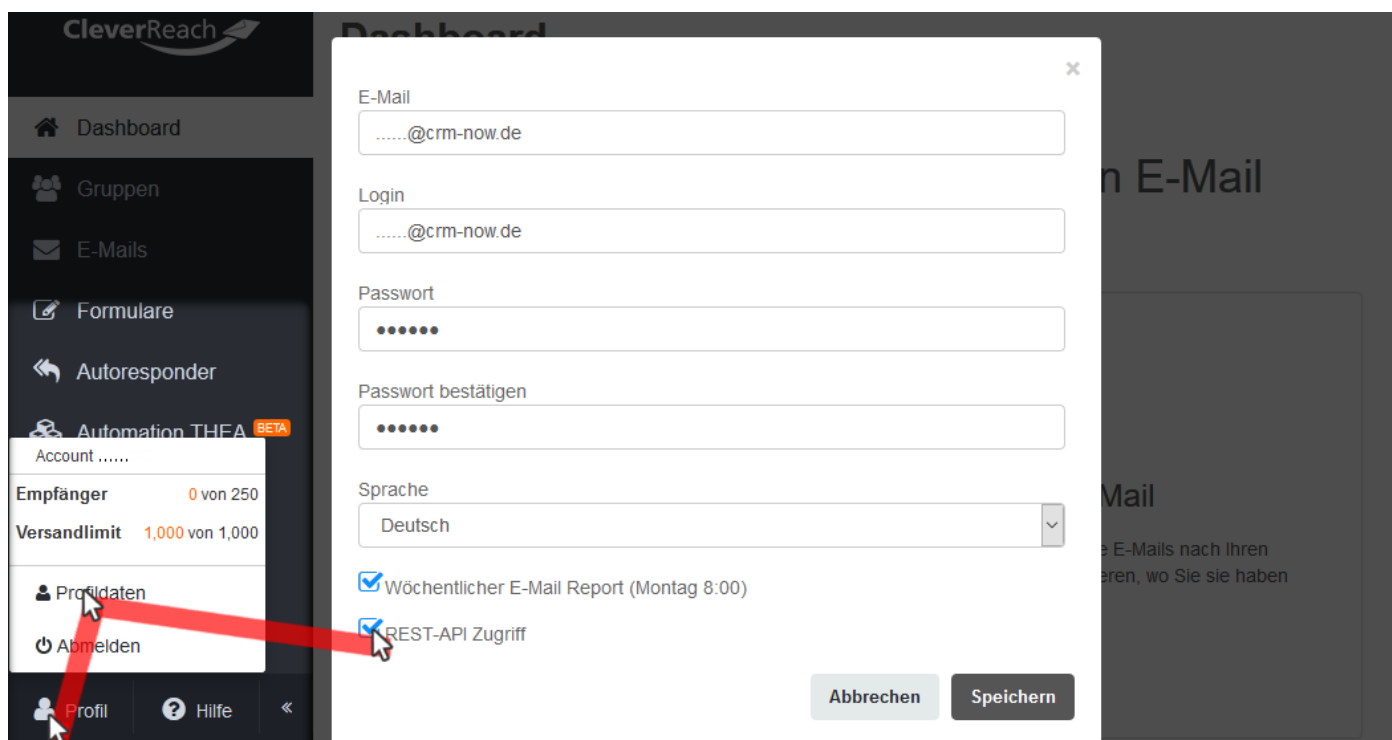
Abbildung 1: REST-API aktivieren
